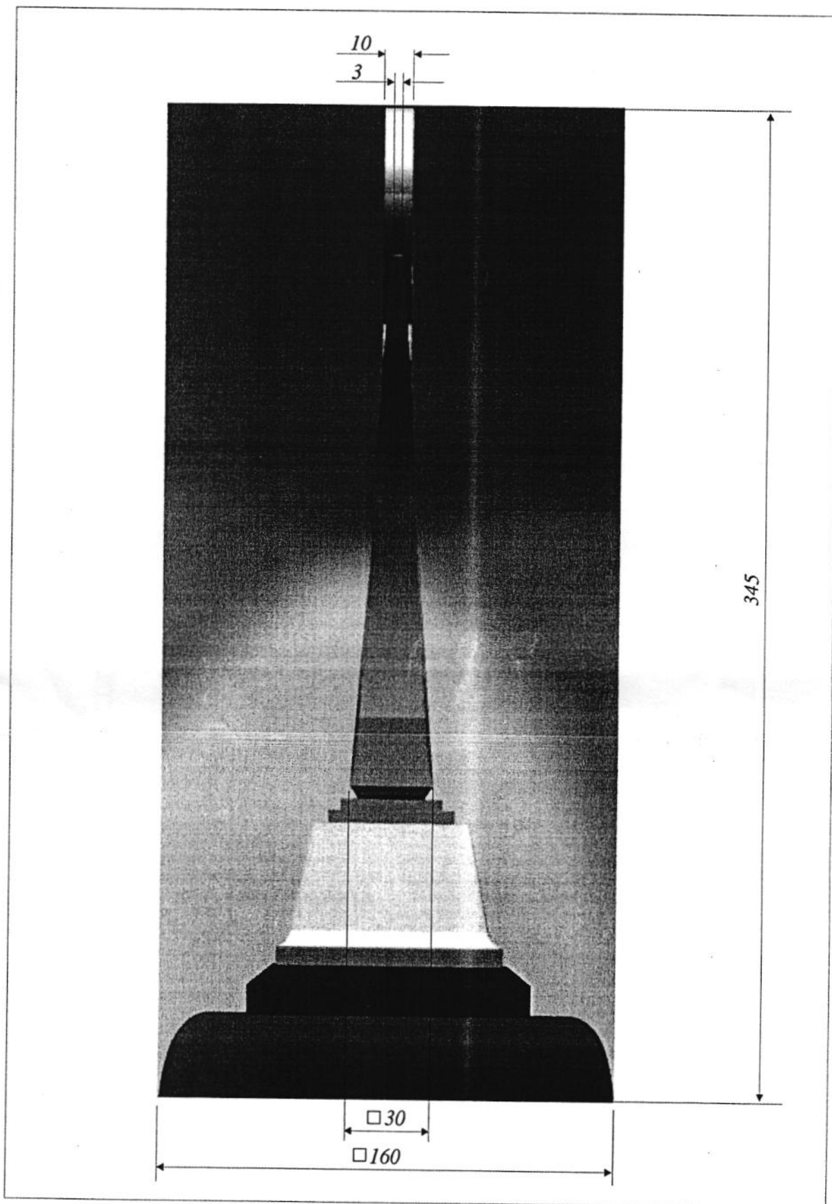
Hình 1.4: Kích thước mặt bên của Cúp Giải thưởng Chất lượng Quốc gia
