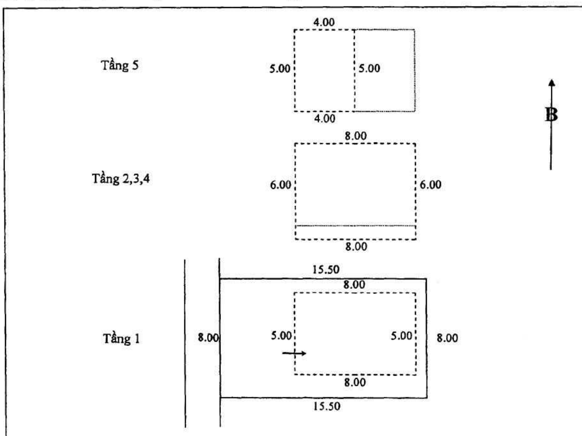
Hình 9 - Sơ đồ nhà 5 tầng có diện tích sàn tầng 1 khác diện tích sàn tầng 2,3,4; diện tích sàn tầng 5 khác với các tầng dưới
